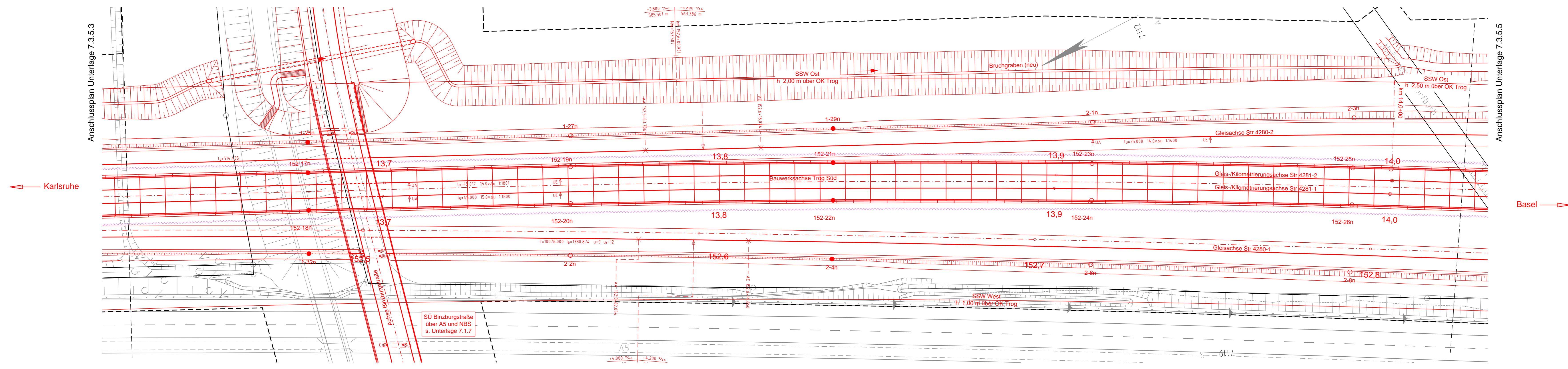
Draufsicht M 1:500
